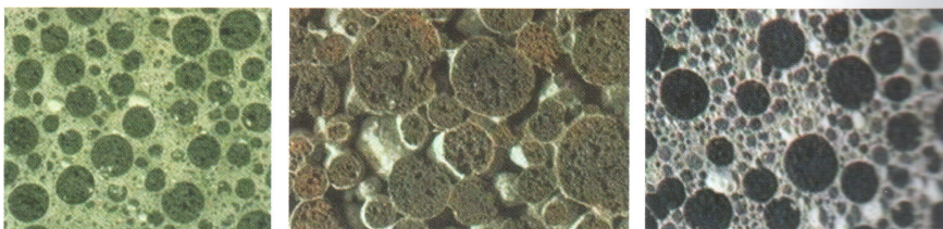
Рис. 1. Структура различных легких бетонов Слева направо: конструкционный легкий бетон (LC) с плотной матрицей; беспесчаный легкий бетон (LAC); беспесчаный легкий бетон с поризованной матрицей (LAC)
