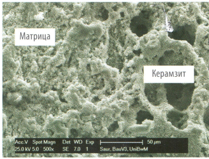
Рис. 6. РЭМ-снимок контактной зоны «матрица — керамзит» в легком бетоне
