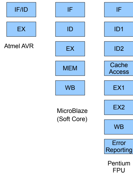
Abbildung 3.11: Einfache Pipelines unterschiedlicher Länge
