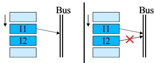
Abbildung 3.4: Wollen zwei Befehle in unterschiedlichen Pipeline-Stufen zur gleichen Zeit auf den Bus zugreifen, kommt es zu einem Struktur-Hazard
